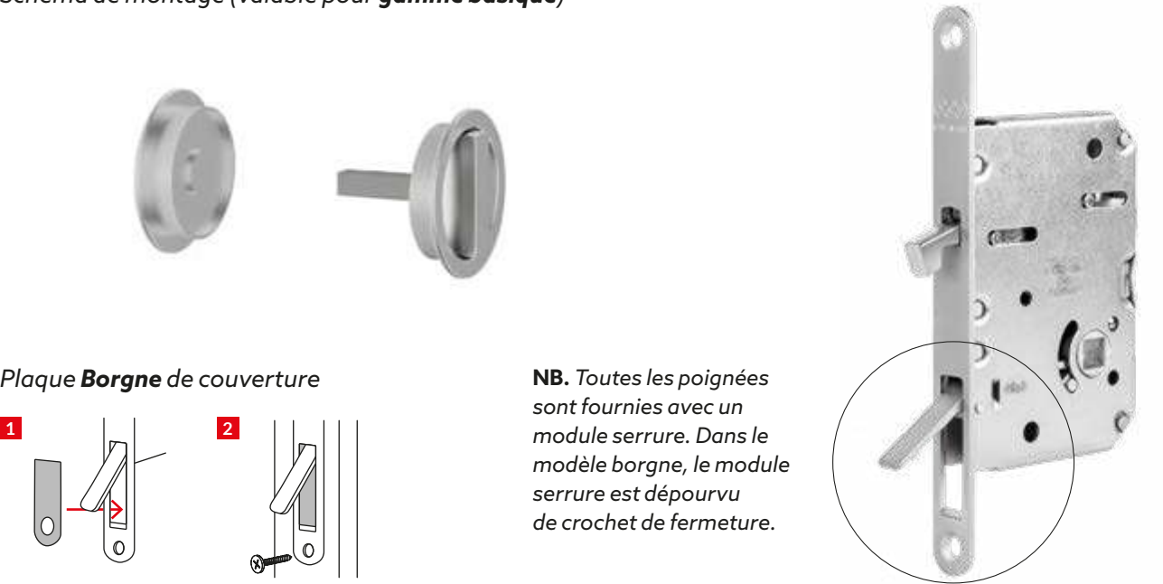
Schéma de montage (valable pour gamme basique )
